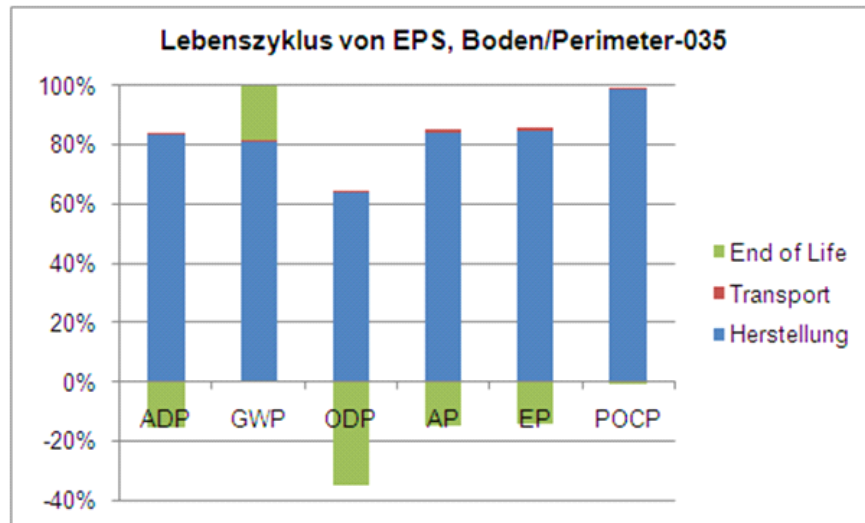
Abbildung 8-5: Lebenszyklus von EPS, Produktuntergruppe Boden/ Perimeter 035
