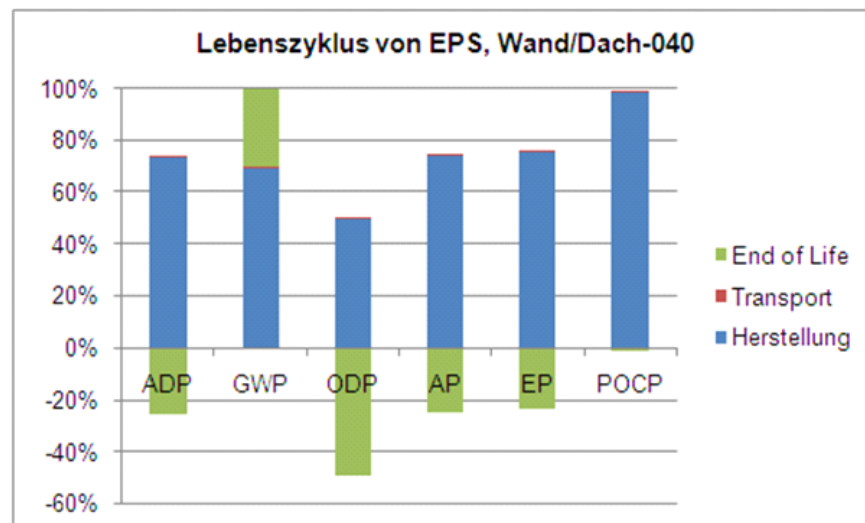
Abbildung 8-6: Lebenszyklus von EPS, Produktuntergruppe Wand/Dach-040
